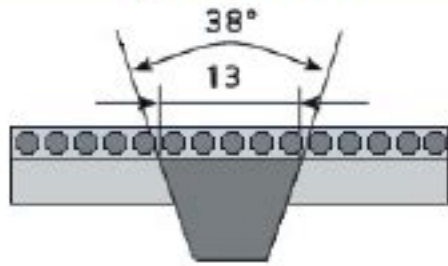
Querschnitt
